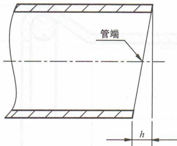
图 1 基管切口斜度
